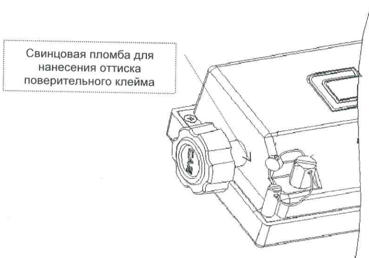
Рисунок А.8 – Схема пломбировки весов складских HFS, R, UFS, CPS (с использованием индикатора NT-200A, NT-200S, NT-201A, NT-201S)
