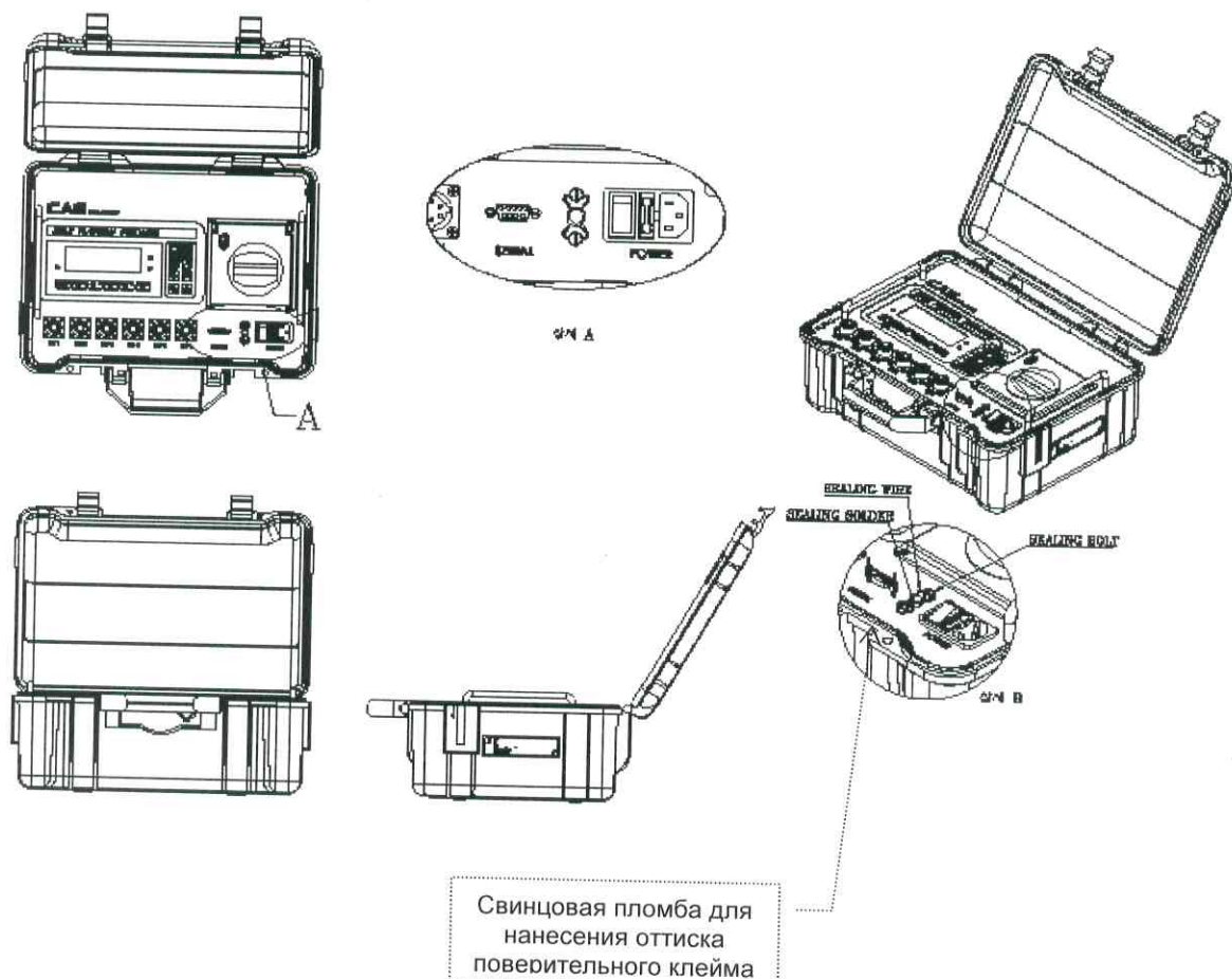
Рисунок А.12 – Схема пломбировки весов складских RW (с использованием индикатора RW-2601P)
