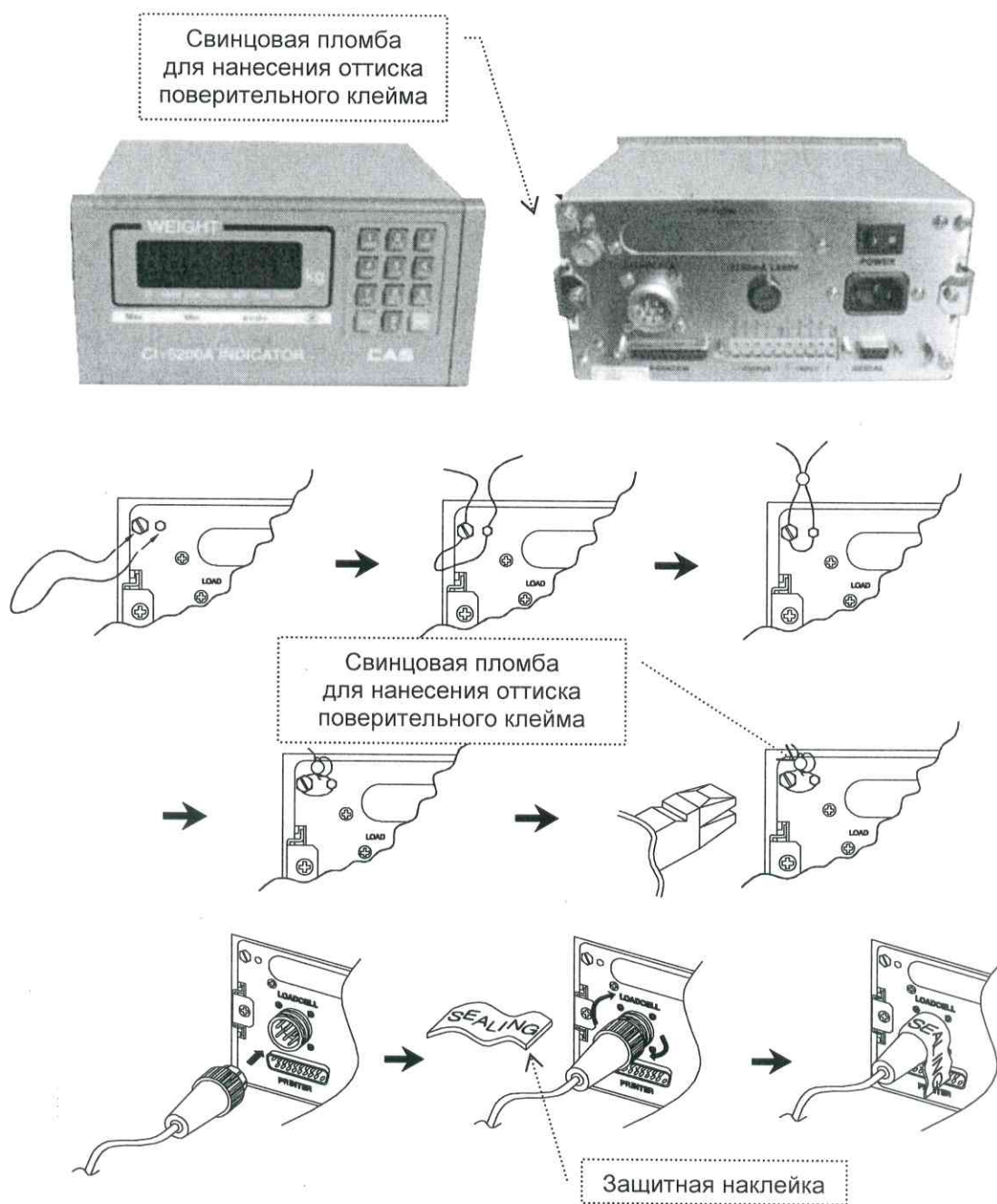
Рисунок А.5 – Схема пломбировки весов складских HFS, R, UFS (с использованием индикатора CI-5010A, CI-5200A)
